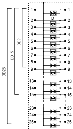
D : Diodo de avalancha
