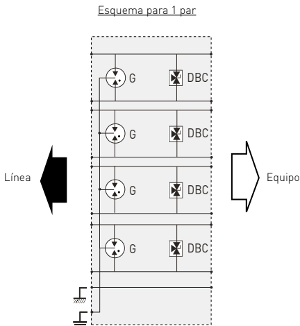
G : Descargador de gas tripolar DBC : 3-pole Diodo baja capacidad
